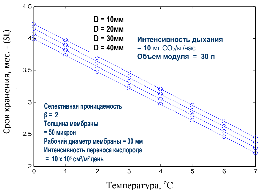
Рис. 3. Сроки хранения яблок в модуле с модифицированной атмосферой в зависимости от температуры при различных рабочих диаметрах мембран
