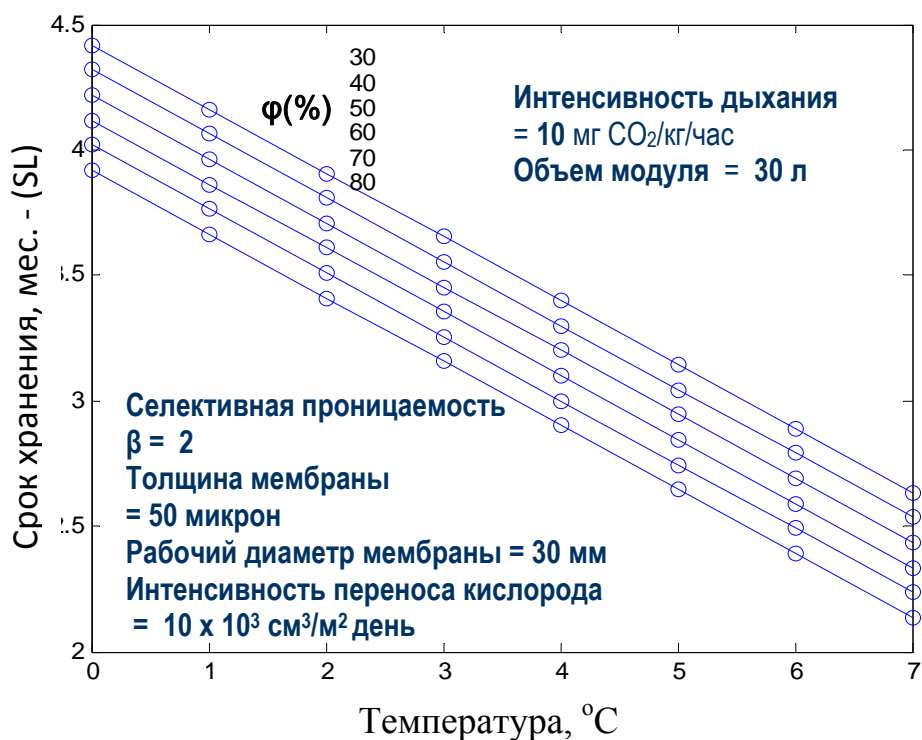
Рис. 2. Сроки хранения яблок в модуле с модифицированной атмосферой в зависимости от температуры и относительной влажности
